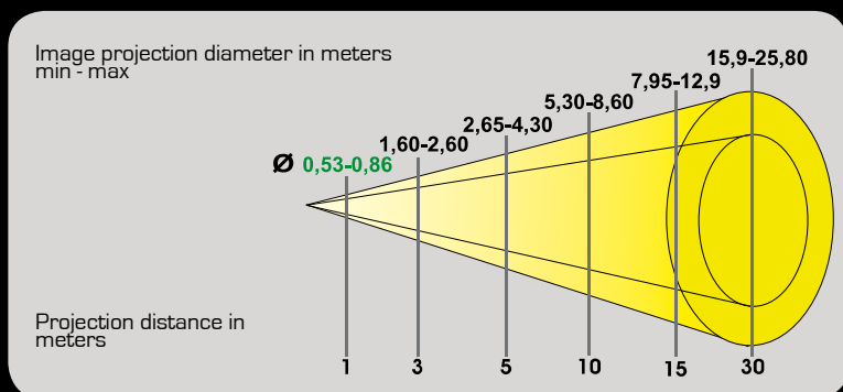
DIMENSIONE DI PROIEZIONE CON EFFETTI DINAMICI
