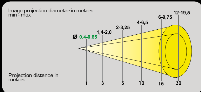
DIMENSIONE DI PROIEZIONE CON GOBO
